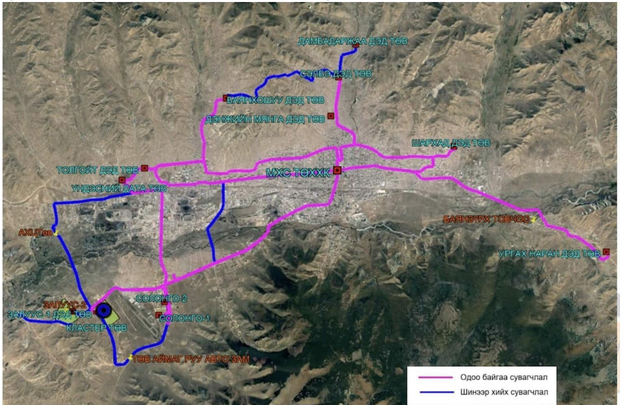
Зураг 5. Улаанбаатар хотын цагирган сүлжээ бүхий сувагчлалын трасс
